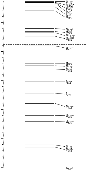
^{136}_{56}\text{Ba}_{80}, p
