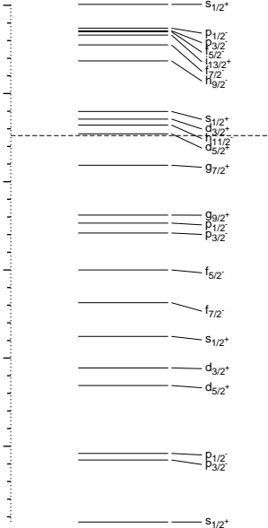
^{146}\text{Sm}_{84}, p
