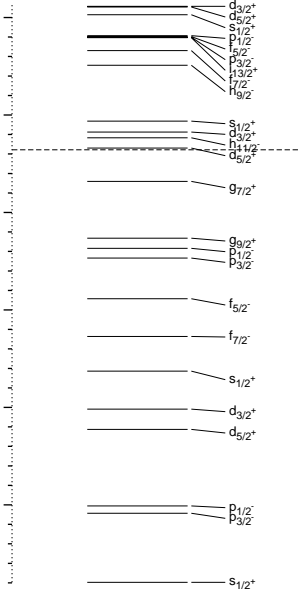
^{142}\text{Sm}_{80}, p
