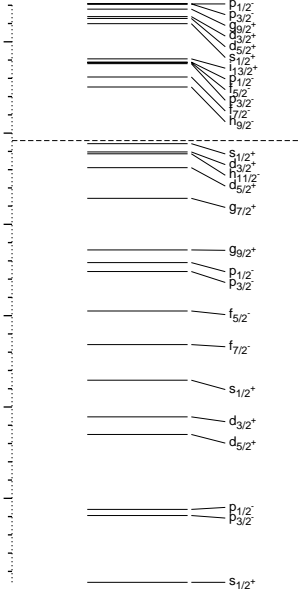
^{142}\text{Sm}_{80}, n
